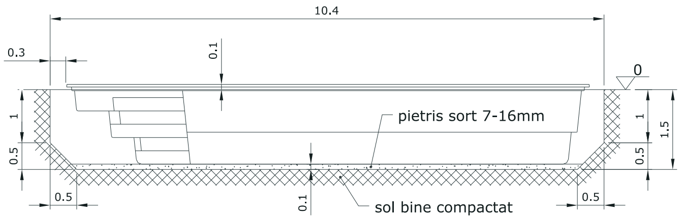
Sectiunea A-A
